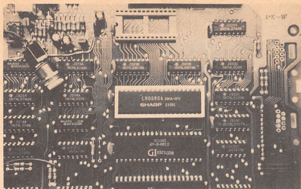
↑白線で囲んだところがZ80Aだ。
