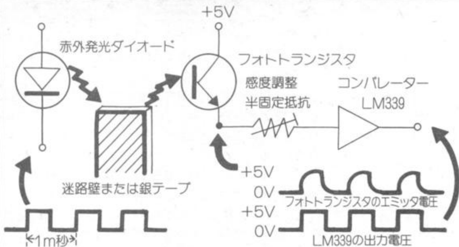
図4 センサ回路
