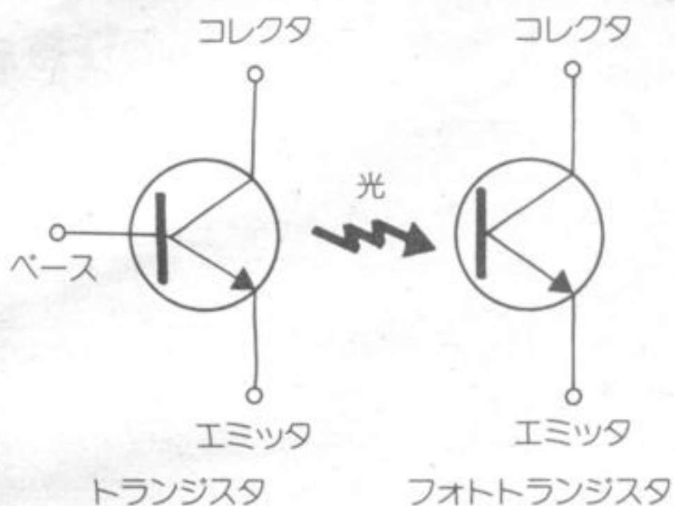
図3 フォトトランジスタ
