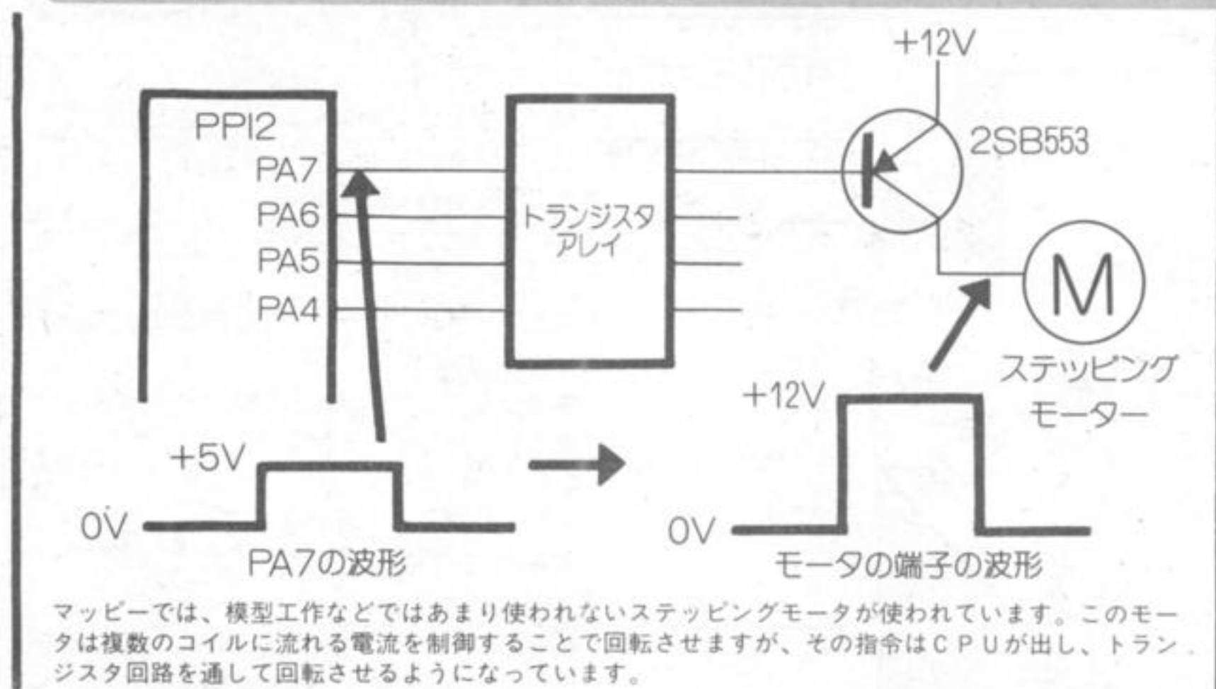
図2 ステッピングモーター駆動回路
