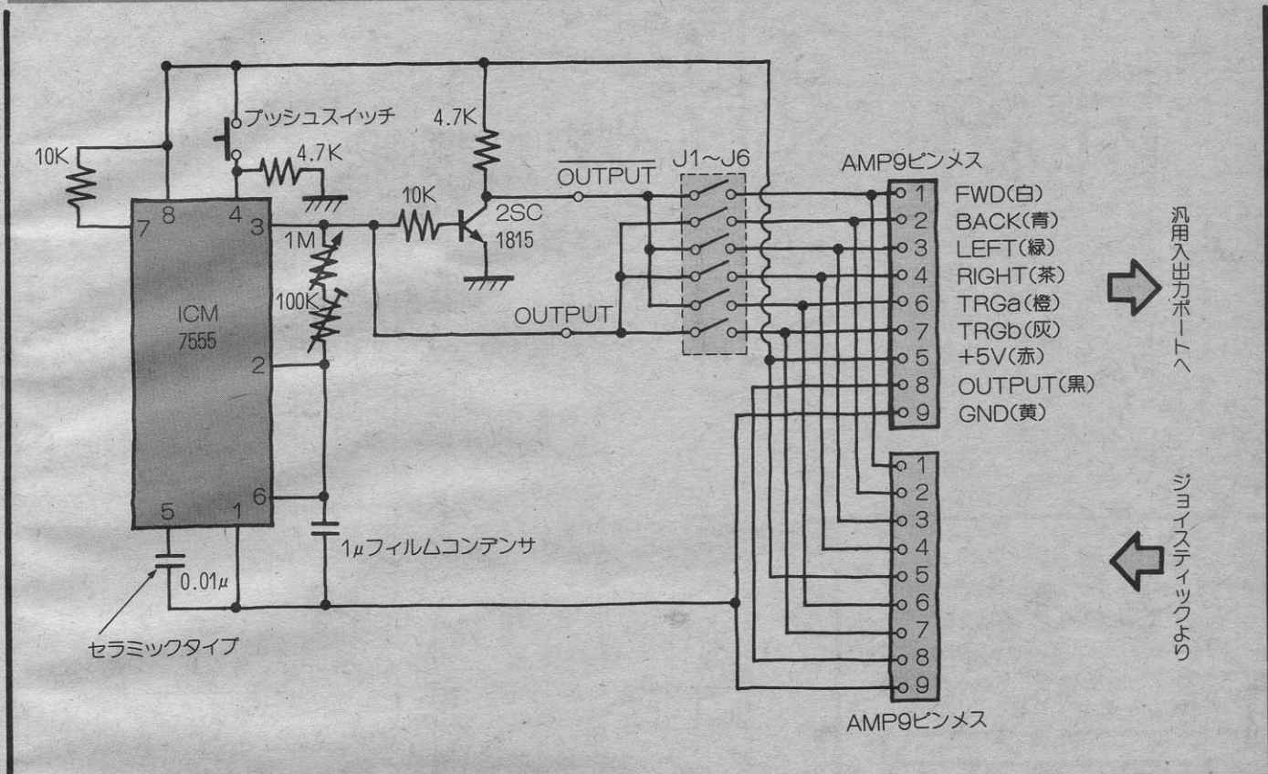
图2 全回路图
