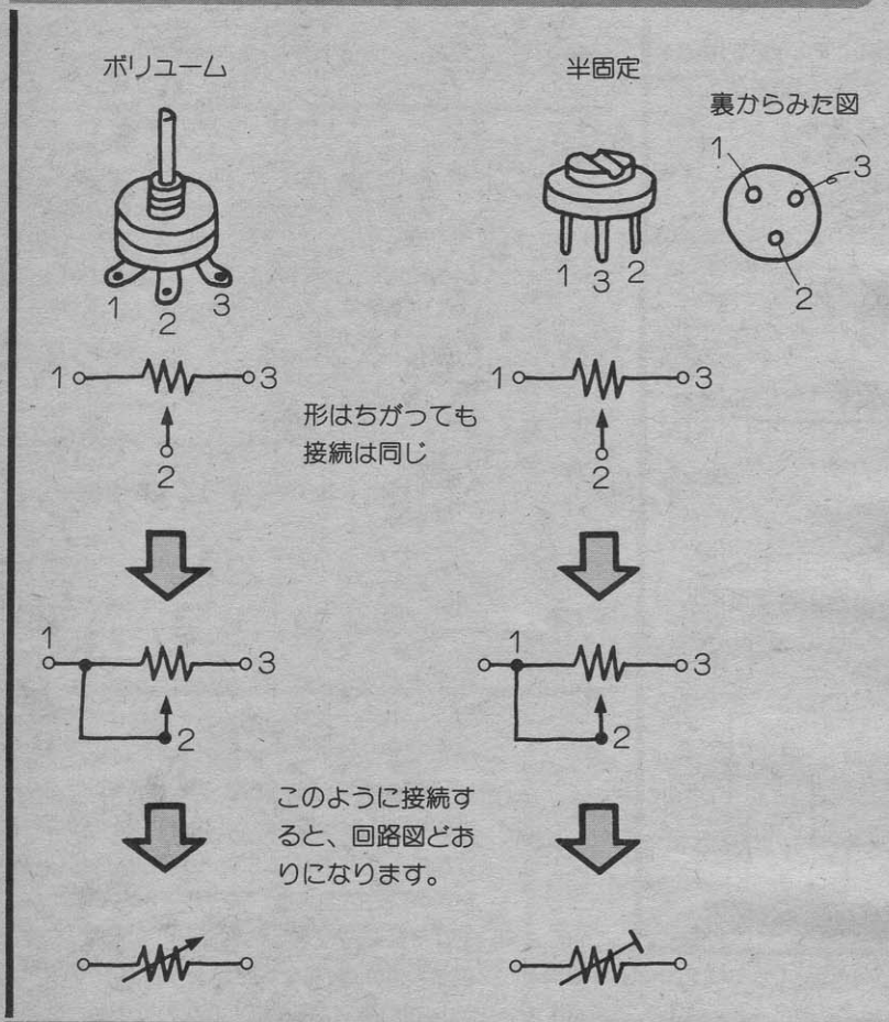
図6 可変抵抗器の接続
