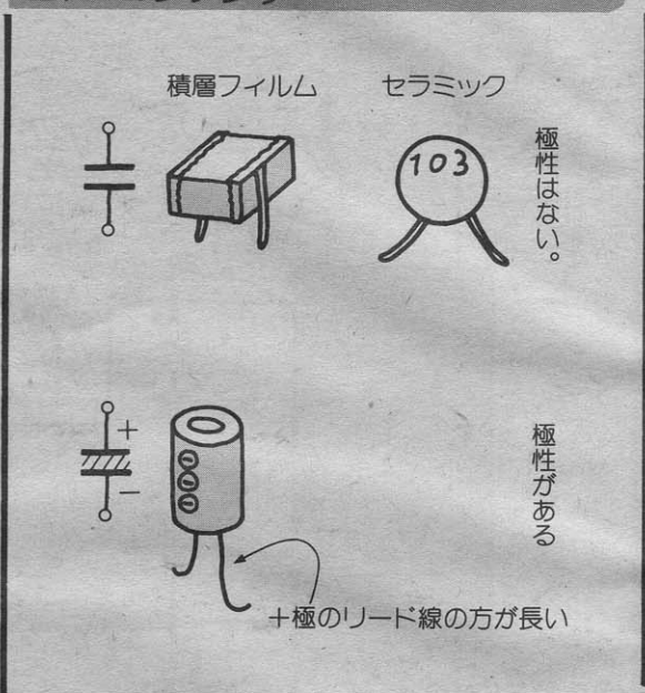
図7 コンデンサ
