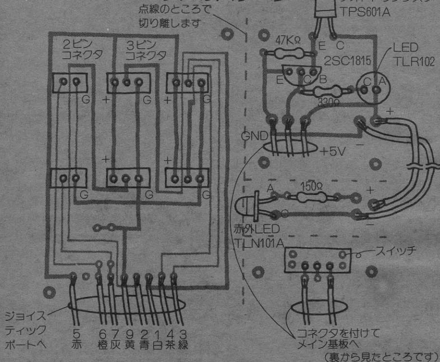
図B ロジックチェッカーのパターン
