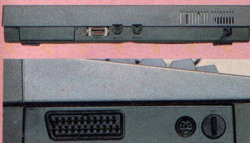
▲ 上がHC-6の背面部。"MONITOR"の表示がコンポジット出力端子。1本のケーブルで映像・音声が出されるけど、先端部は2本に分かれていて、モニタの映像、音声入力端子に接続されるようになっている。
