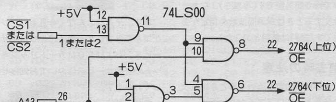
図4 2764を2個連続して配置する追加回路
