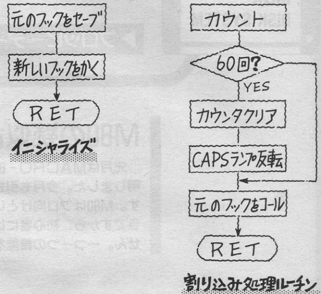
図12 CAPSランプ点滅のフローチャート
