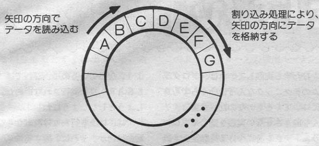
● 図1 リングバッファ
