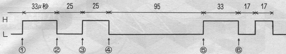
▶ 図1 マウス・トラックボールのタイミング
