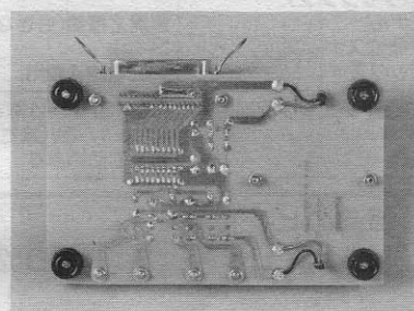
写真2 コントロール基板の裏側
