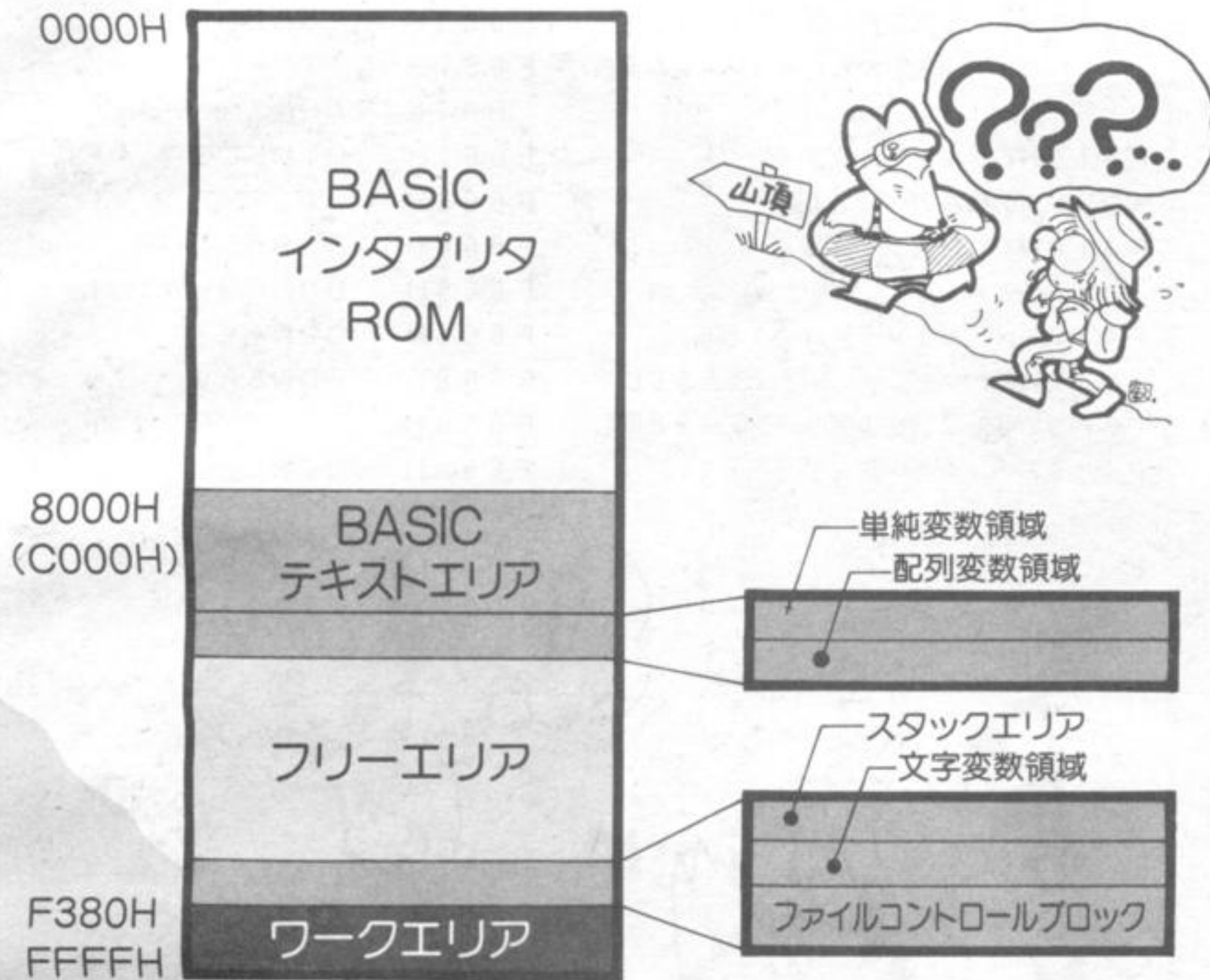
▲図1 MSXのメモリマップ
