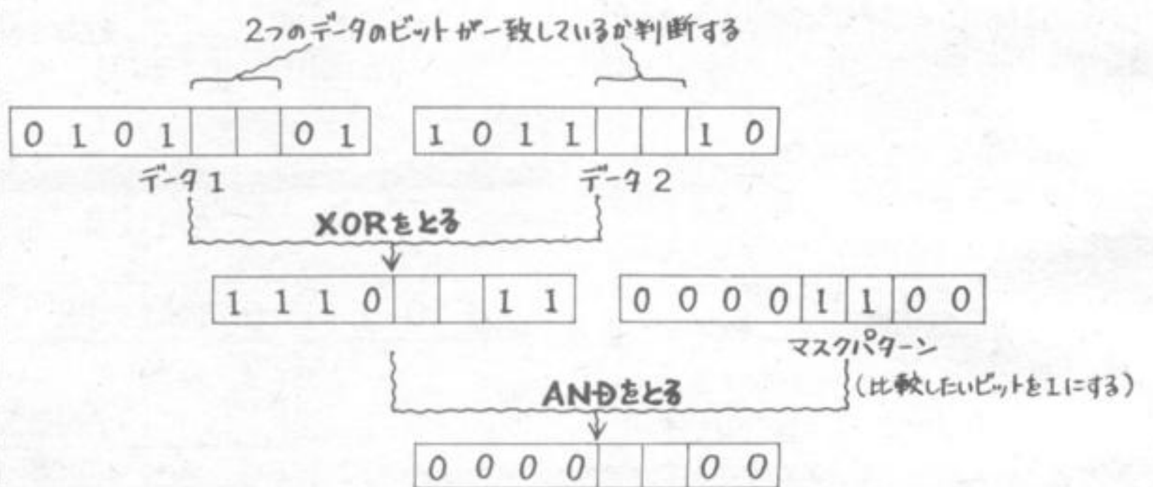
▶ 図6 XOR命令を使って、ビットの一致を確認する。
