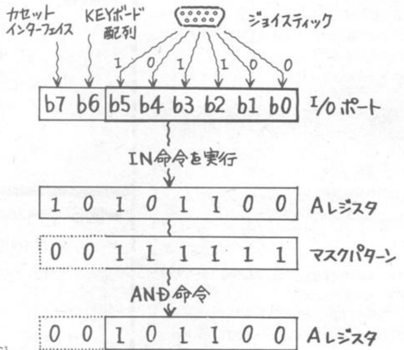
AND命令を使って、必要なビット情報が取り出せる
