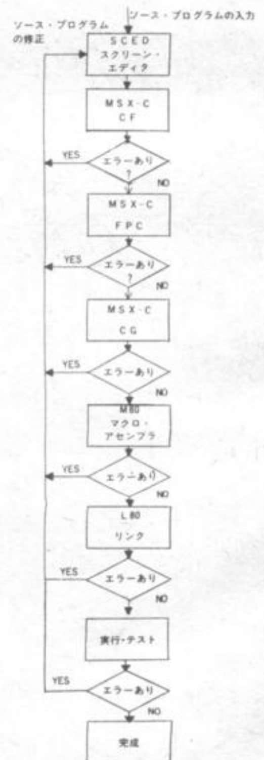
図1 MSX-Cのプログラム開発手順
