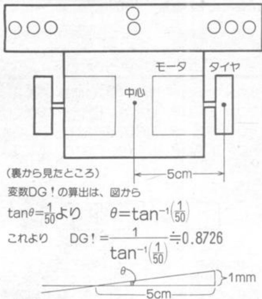
図1 回転角度の算出
