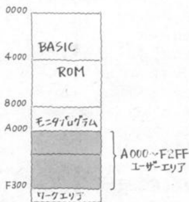
32k,64k MSX メモリマップ
