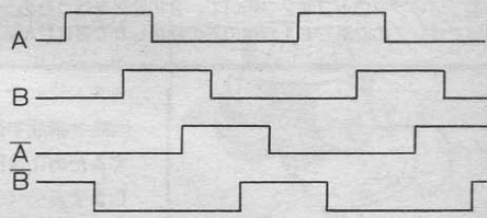
(c) 1～2相励磁
