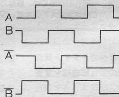
(b) 2相励磁
