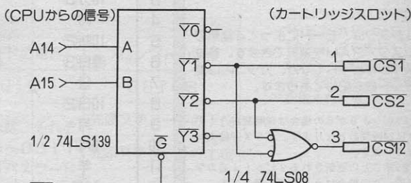
図B CS信号の作成例
