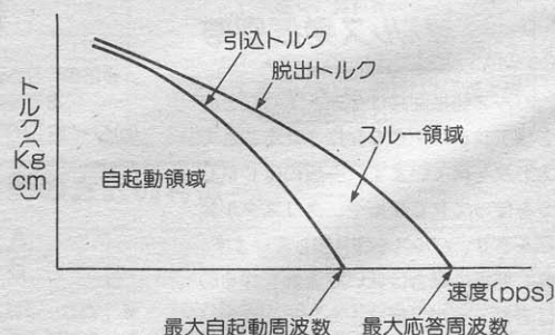
図14 トルク・スピード特性
