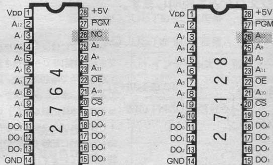
図A 2764と27128のピン接続
