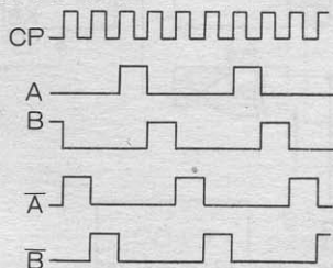
(b) タイミングチャート
