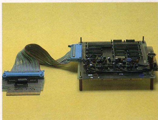
◆12月号で紹介したビデオスキャナーの基板だ。これを作るには、かなりの技術が必要だけど。
