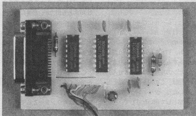
▲取り付けた部品を真上からみたところです。下の図3と比較して、確認してください。
