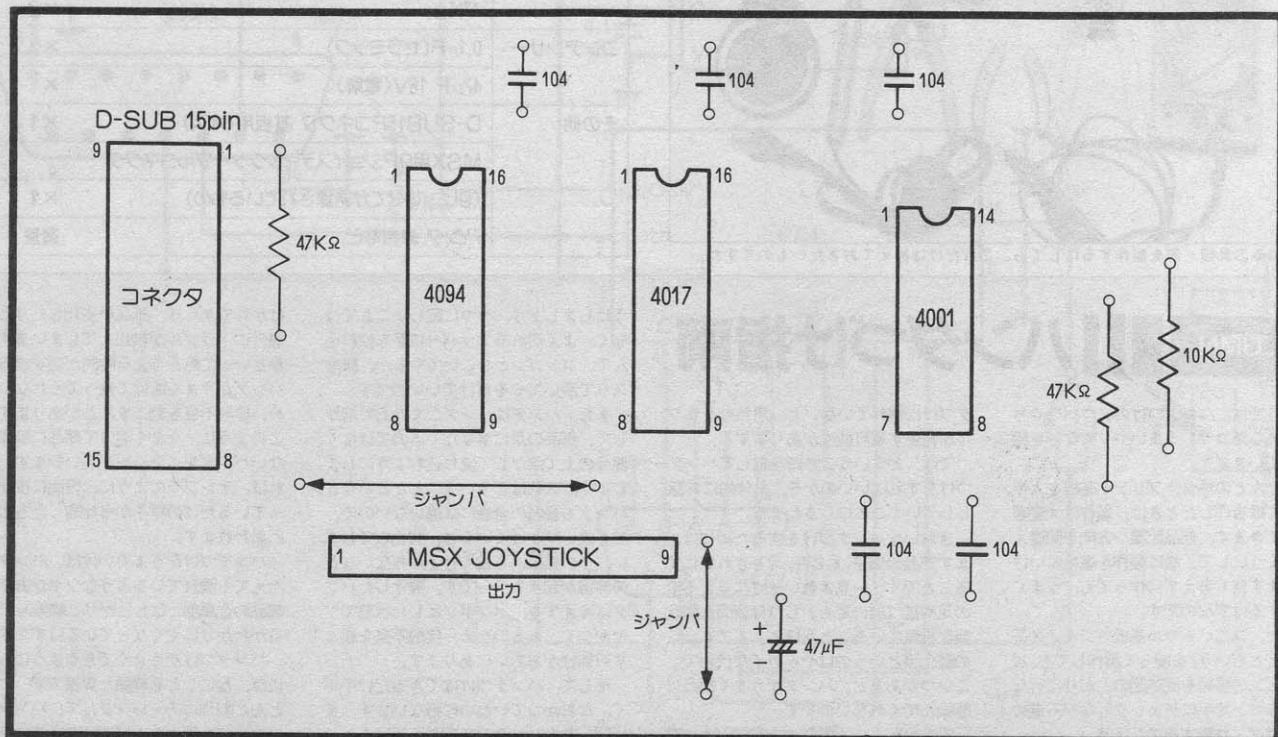
図3 部品配置図
